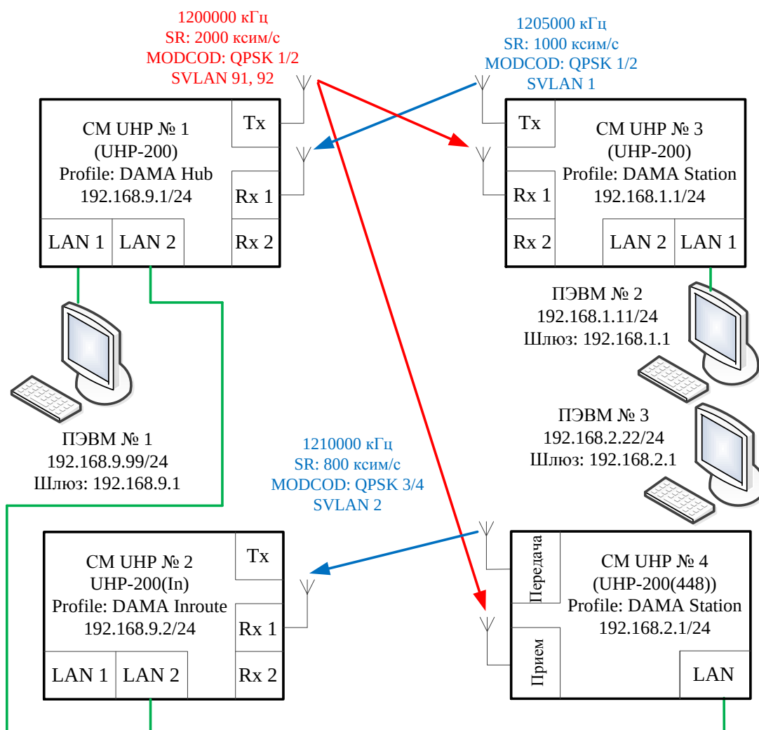
Рисунок 4. Сеть топологии «звезда» (DAMA/SCPC)
